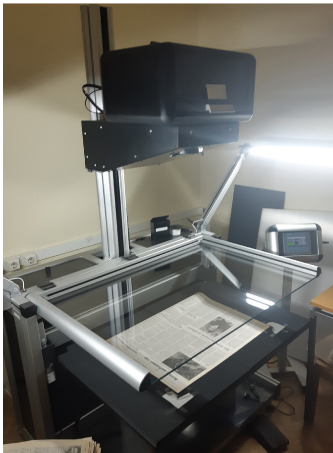
Микрофильмирующая камера ЭЛАР МФ 2002-А1
