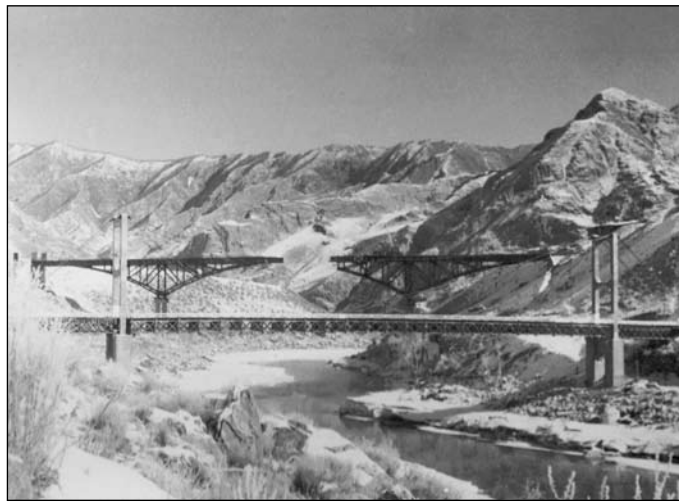
Монтаж конструкций в среднем пролете моста.
